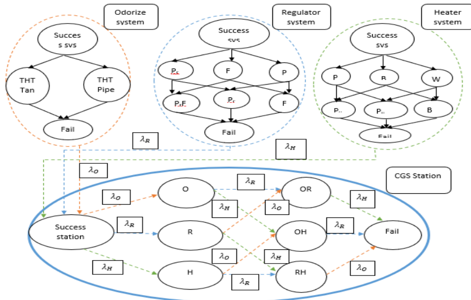
شکل ۱۲: رویکرد سیستماتیک بر اساس مدل مارکوف برای ایستگاه تقلیل فشار
