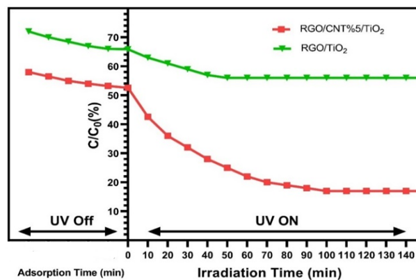
شکل ۹: نمودار روند تجزیه فتوکاتالیستی بخارات تولوئن توسط ایزوپروپانول در غلظت ۲۰ ppm
