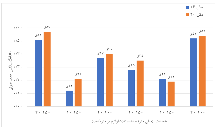
شکل ۶: مقادیر SAA نمونه‌های مش ۱۶ و ۲۰ بر اساس روش RSM (optimized samples) بر حسب دانسیته و ضخامت
