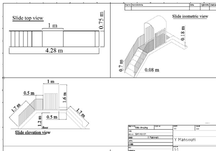
شکل ۷. نقشه طراحی سرسره بر اساس داده های آنترپومتریک کودکان از نماهای مختلف
