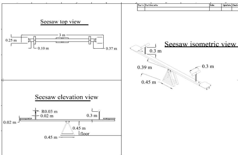
شکل ۳. نقشه طراحی الاکلنگ بر اساس داده های آنتروپومتریکی کودکان از نماهای مختلف
