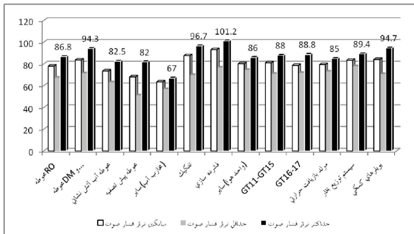
شکل ۱: نتایج اندازه گیری نواز فشار صوت (dB A) در بخش های مختلف مجتمع
