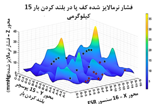
شکل ۴: نمودار سه بعدی فشار نرمالایز شده کف پای راست و چپ در بلندکردن بارهای ۷.۵ و ۱۵ کیلوگرمی. ستاره مشکی (★) اشاره به همبستگی معنادار بین میانگین فشار وارده به ناحیه کمری با میانگین فشار وارده به کف پا و ستاره قرمز (★) اشاره به همبستگی معنادار بین میانگین شاخص بلندکردن بار با میانگین فشار وارده به کف پا دارد.
