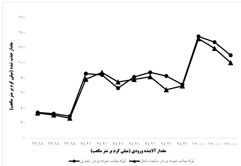
شکل ۴: مقدار جاذب لوله های جاذب نمونه بردار ساخت داخل و نوع تجاری در تراکم های مختلف از تولوئن
