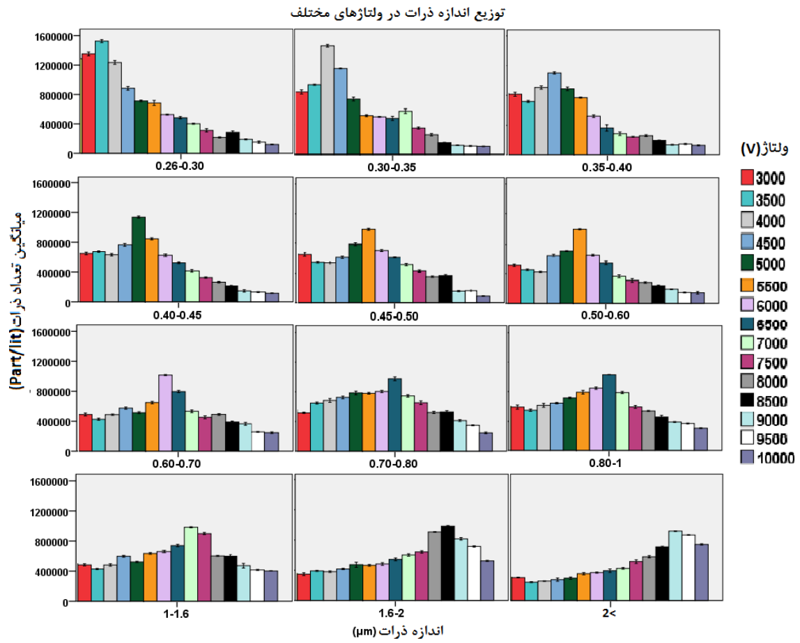
شکل ۳. توزیع اندازه ذرات خروجی از دستگاه DMA در ولتاژهای مختلف
