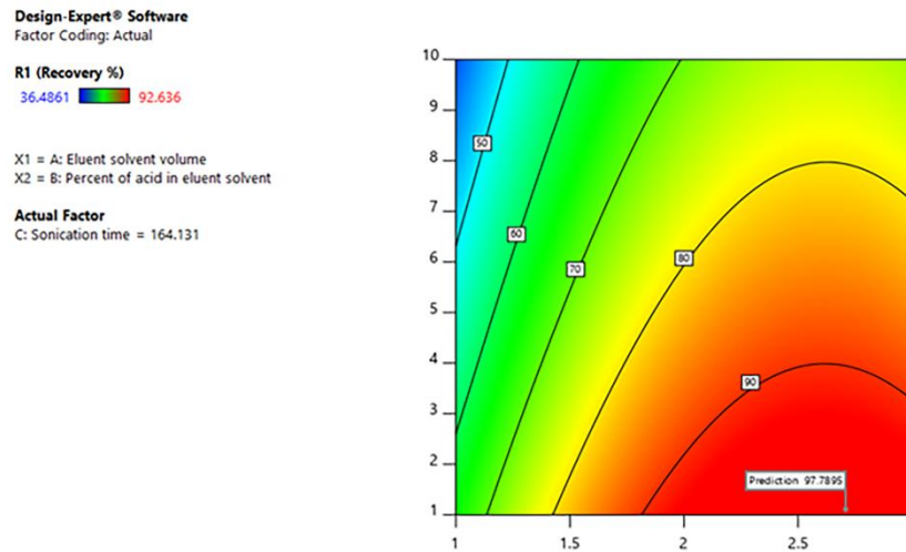
شکل ۳. رابطه متقابل حجم حلال شویش، مقدار اسید و مدت زمان بازیافت ثابت ۱۶۴/۱۳۱ ثانیه با میزان بازیافت بنتازون
