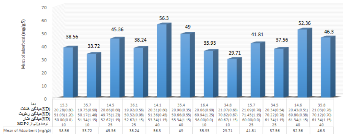
نمودار ۵: میانگین میزان جذب H_2S در غلظت ۲۰ ppm از جاذب AC/MOF-5 در درصدهای مختلف وزنی و تاثیر فاکتورهای دما، رطوبت و فشار
