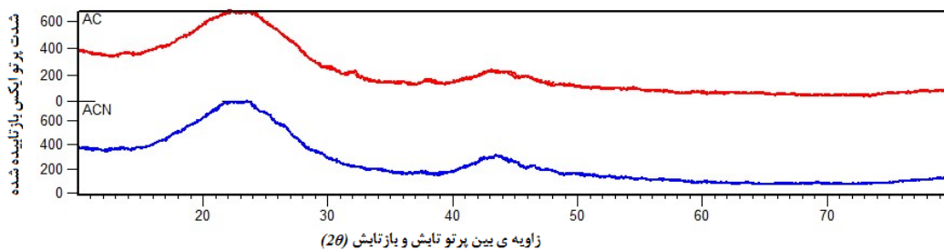
شکل (۲) - الگوهای پراش اشعه ایکس جاذب های زغال فعال (AC) و زغال اصلاح شده با اسید (ACN)
