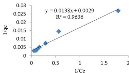
شکل ۶. ایزوترم لانگمیر در جذب زایلن بر روی جاذب کربن اکتیو
