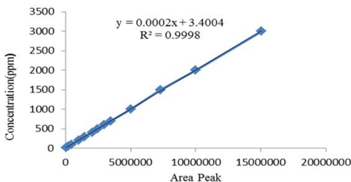
شکل ۱. منحنی کالیبراسیون زایلن
