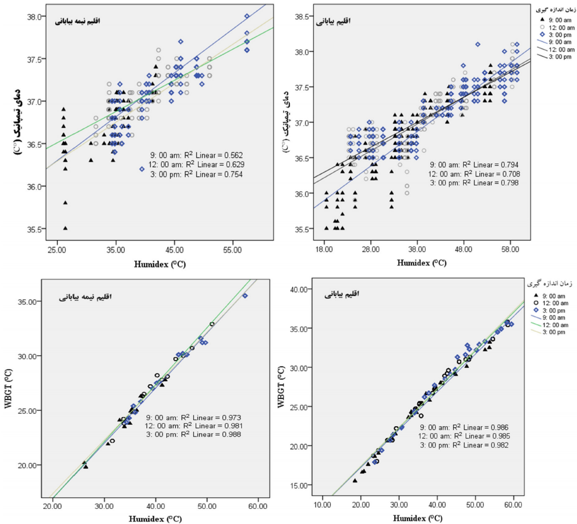
شکل ۱: بررسی هم‌بستگی شاخص Humidex با شاخص WBGT و پاسخ فیزیولوژیک دمای پرده سماخ در نواحی بیابانی و نیمه بیابانی و در ساعات مختلف روز (ساعت ۹، ۱۲، و ۳ عصر)
