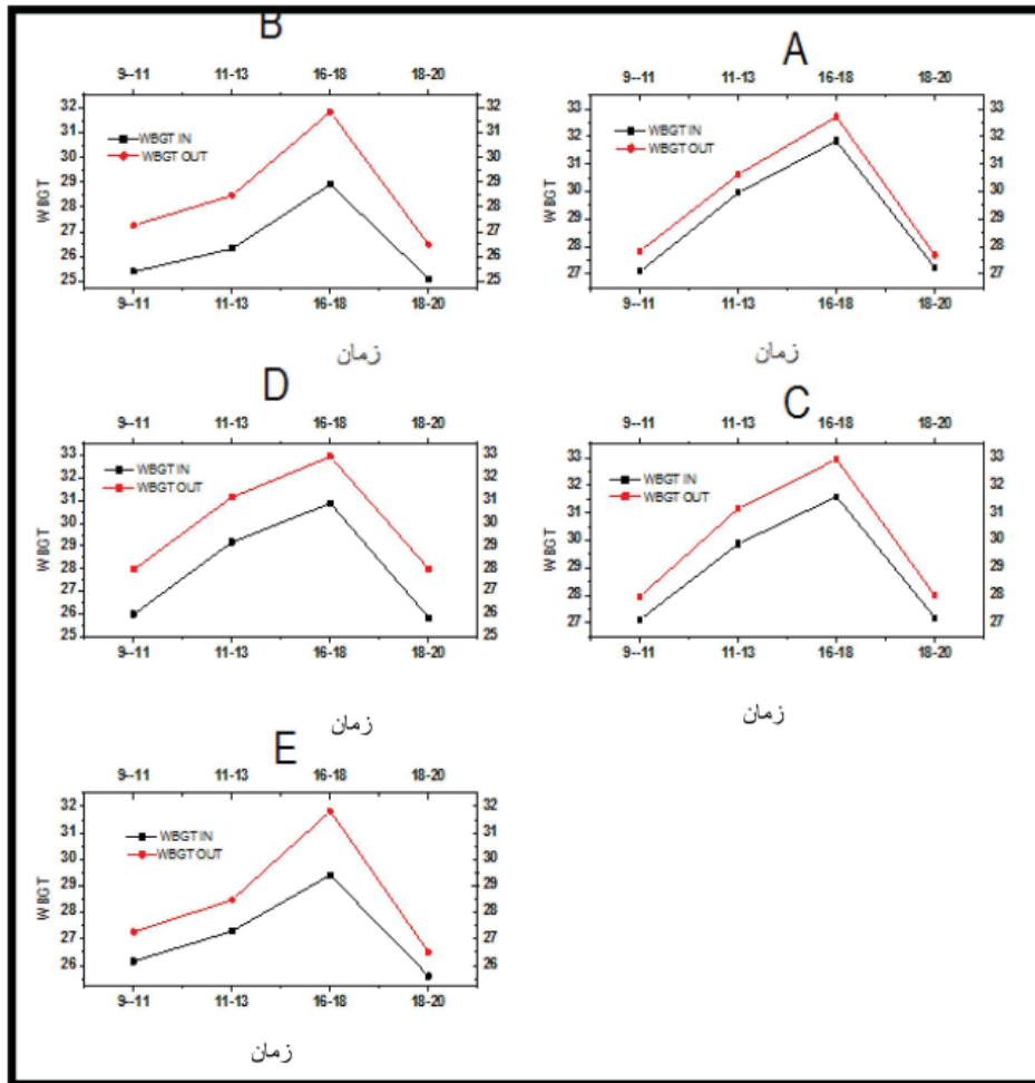
شکل ۲: تغییرات میزان WBGT در ساعات مختلف روز کاری در کارگاه‌های مختلف، A: کارگاه‌های صافکاری B: کارگاه‌های درب و پنجره سازی آلومینیومی C: کارگاه‌های نقاشی D: کارگاه‌های مکانیکی و E: کارگاه‌های جوشکاری
